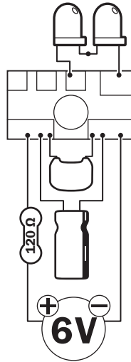
7 Einzelblinker mit 2 LEDs Flasher with 2 LEDs
