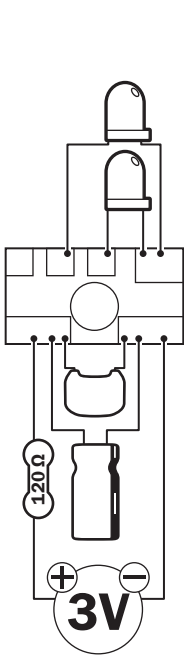
4 Wechselblinker mit 1 LED pro Kanal für 3 V Alternating Flasher with 1 LED per channel for 3 V
