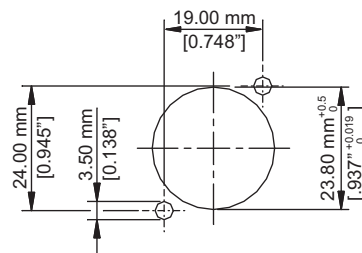
Frontplattenausschnitt (Rückseite) Panel Cutout (Rear Side)
