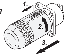
Aussteck-Vorgang Separation
